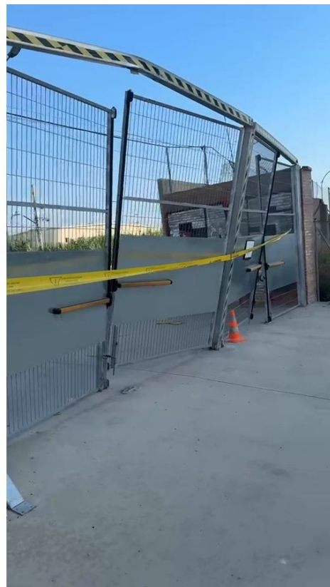
Fotografies 4 i 5 (fotogrames del vídeo Accés_NdT.mp4). Esquerra: fulla tancada provisionalment amb cadena, barra antipànic existent i muntant desplomat amb tornapunta. Dreta: pòrtic superior deformat i fulles fora de pla.
